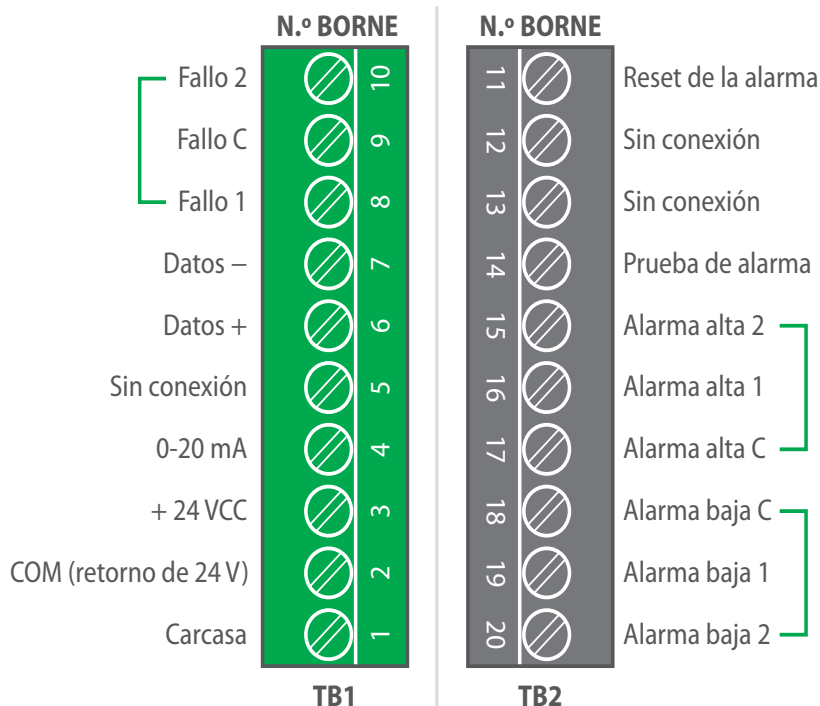
Fig. 16 Terminales de campo
