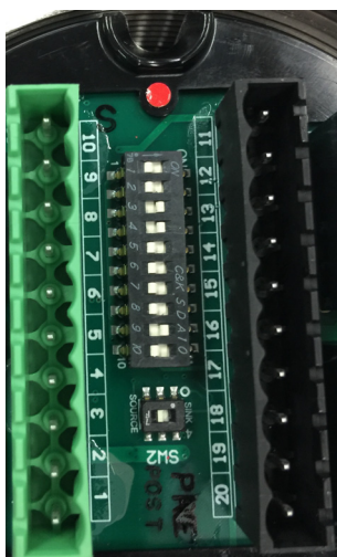
Fig. 17 Ubicación del interruptor DIP
