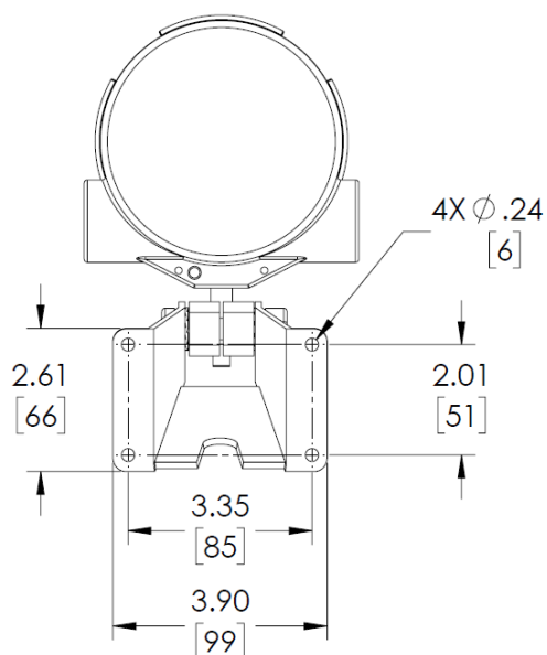
Fig. 13 FL500 y soporte de montaje, vista posterior
