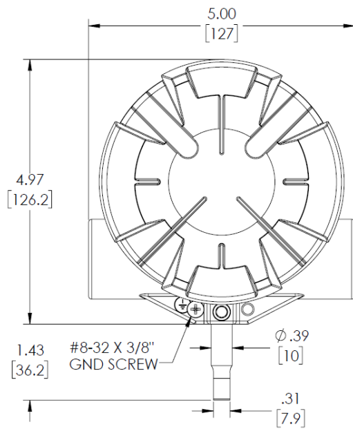
Fig. 9 Plano acotado del FL500, vista frontal
