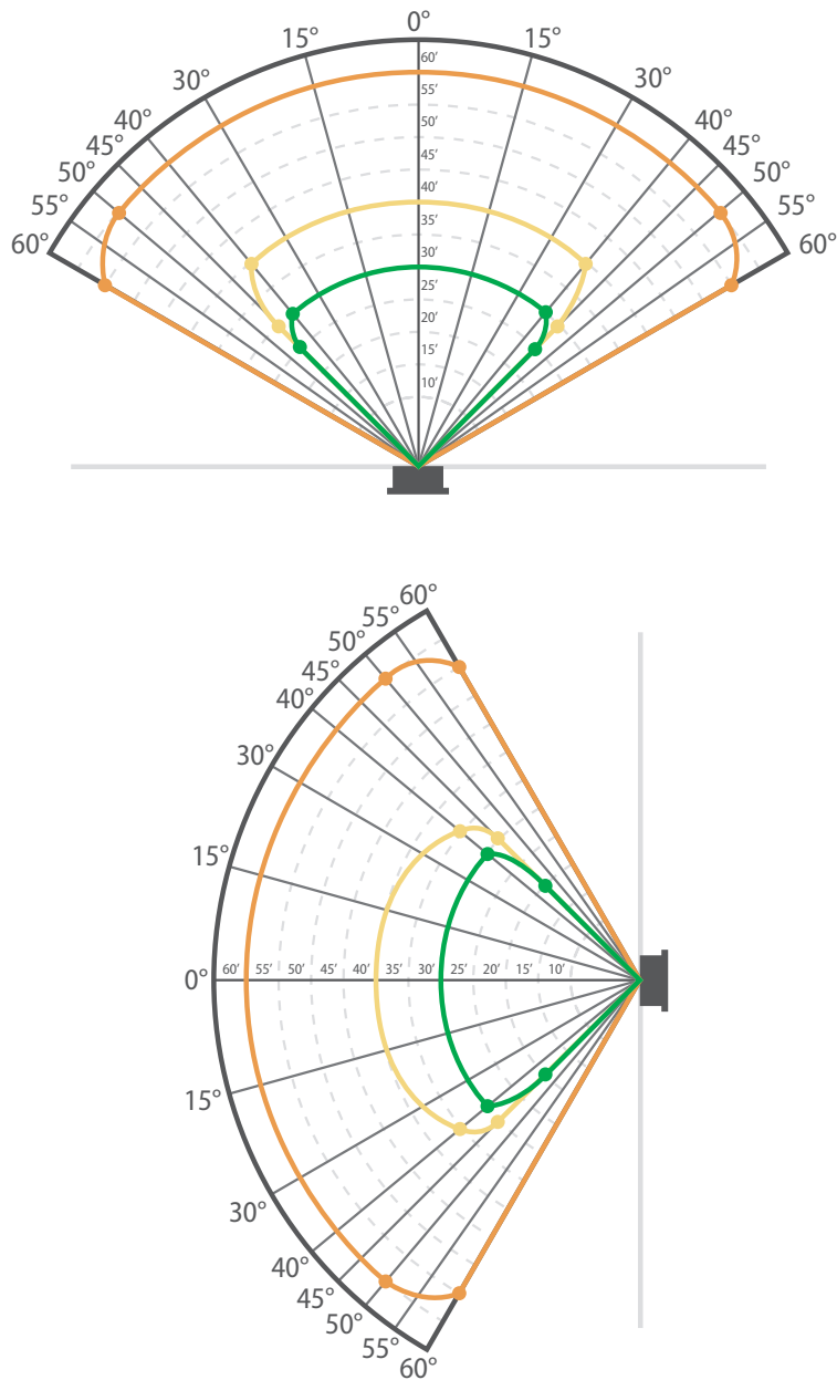
Fig. 7 Campo de visión de etano
