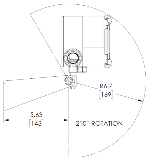
Fig. 11 FL500 y soporte de montaje, vista lateral
