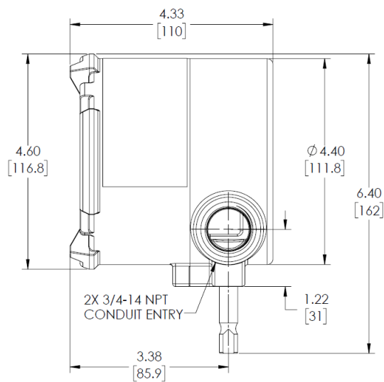
Fig. 10 Plano acotado del FL500, vista lateral
