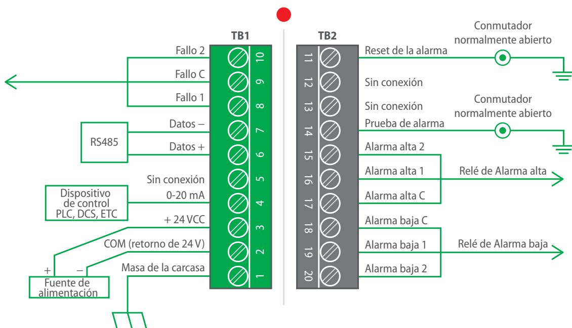
Fig. 15 Diagrama de cableado
