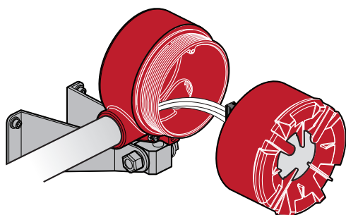
Fig. 14 Carcasa y base del FL500
