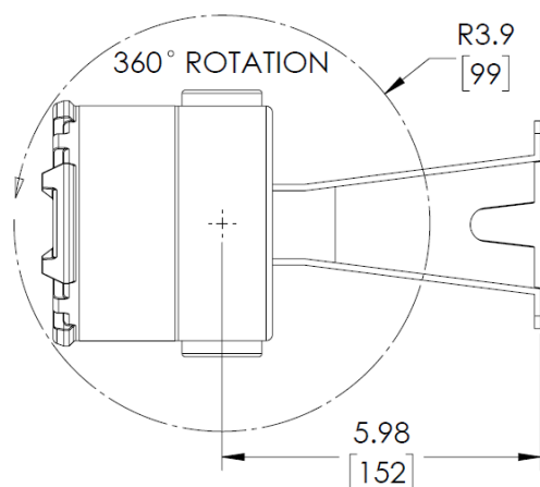
Fig. 12 FL500 y soporte de montaje, vista en planta
