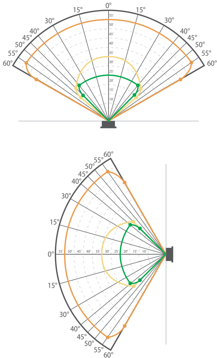
Fig. 8 Campo de visión de butano
